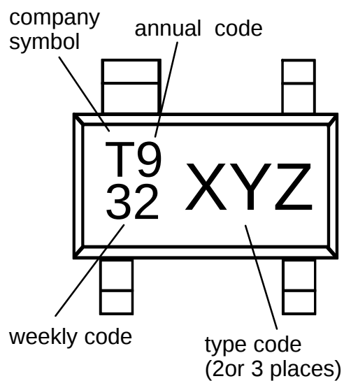
SOT343R
