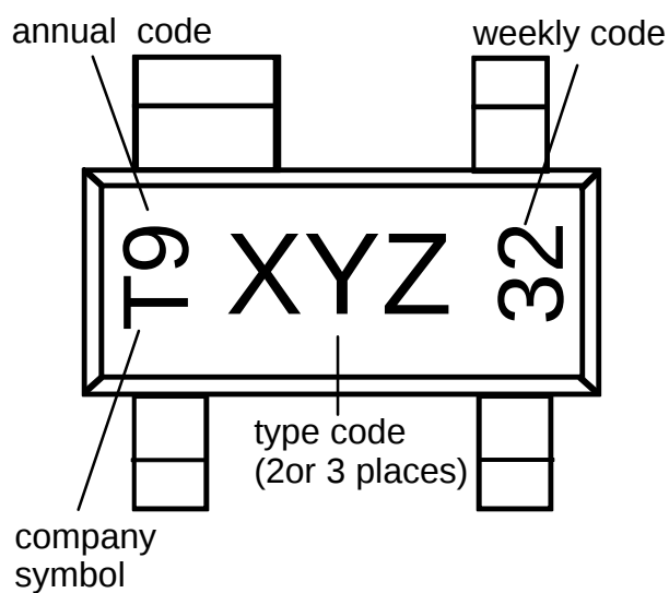
SOT143R
