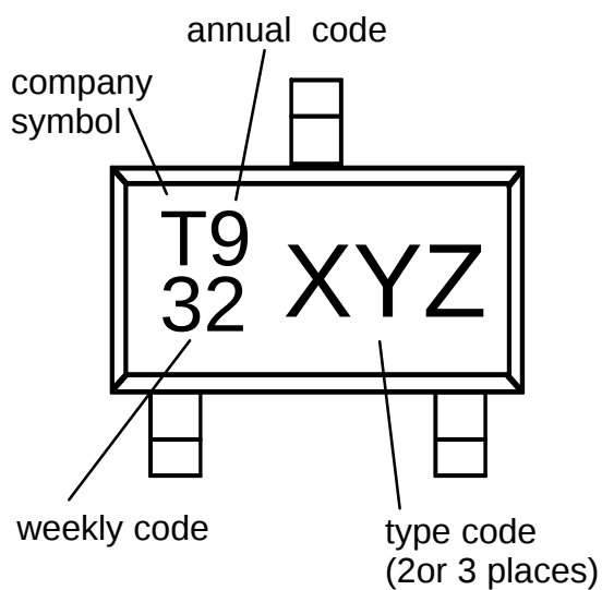
SOT323
