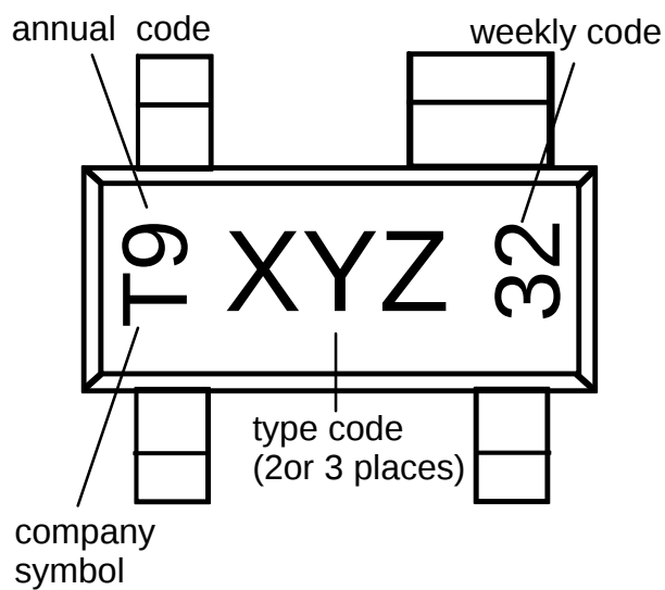
SOT143
