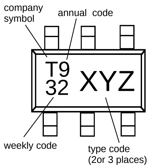
SOT363
